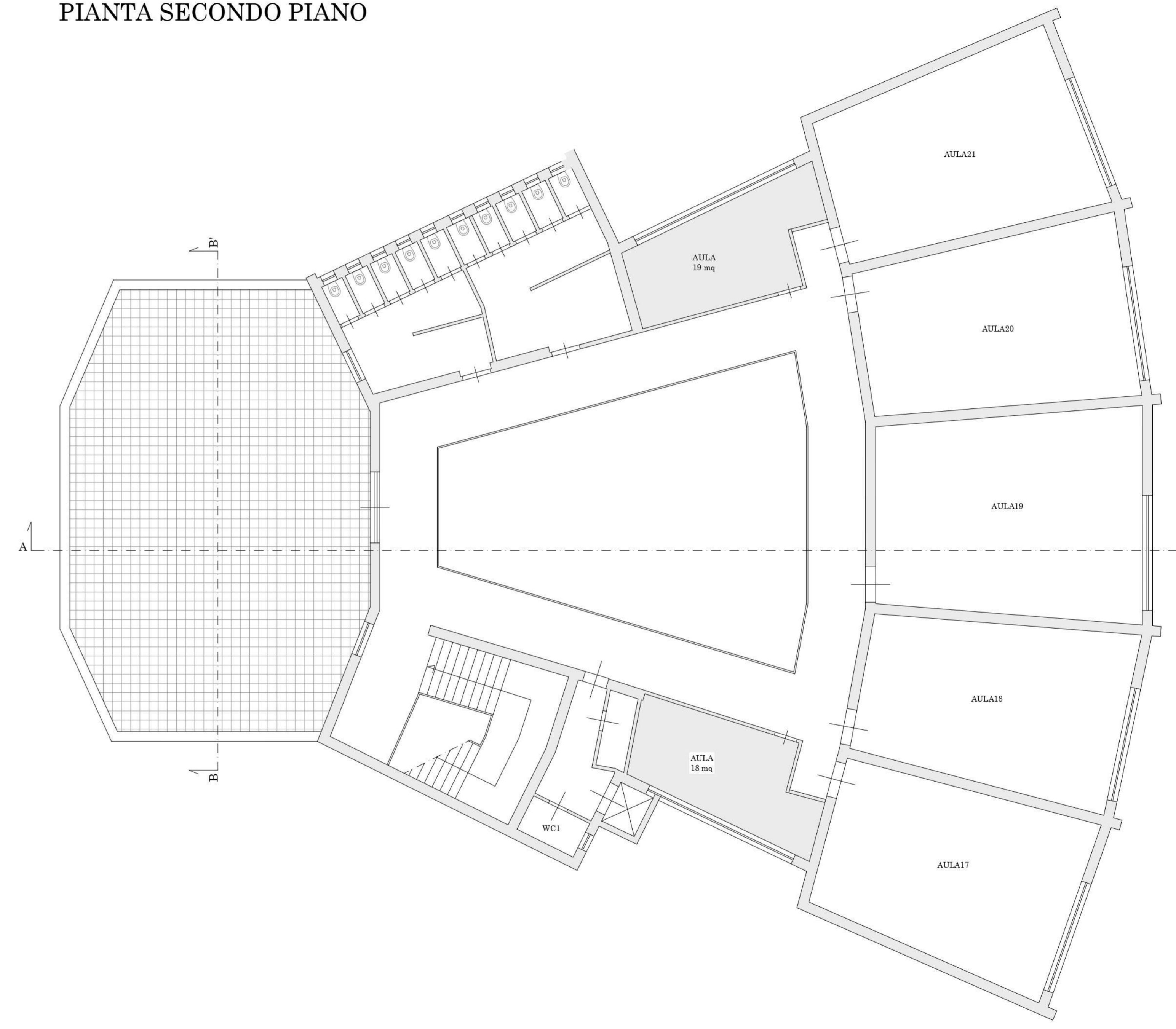
PIANTA SECONDO PIANO
